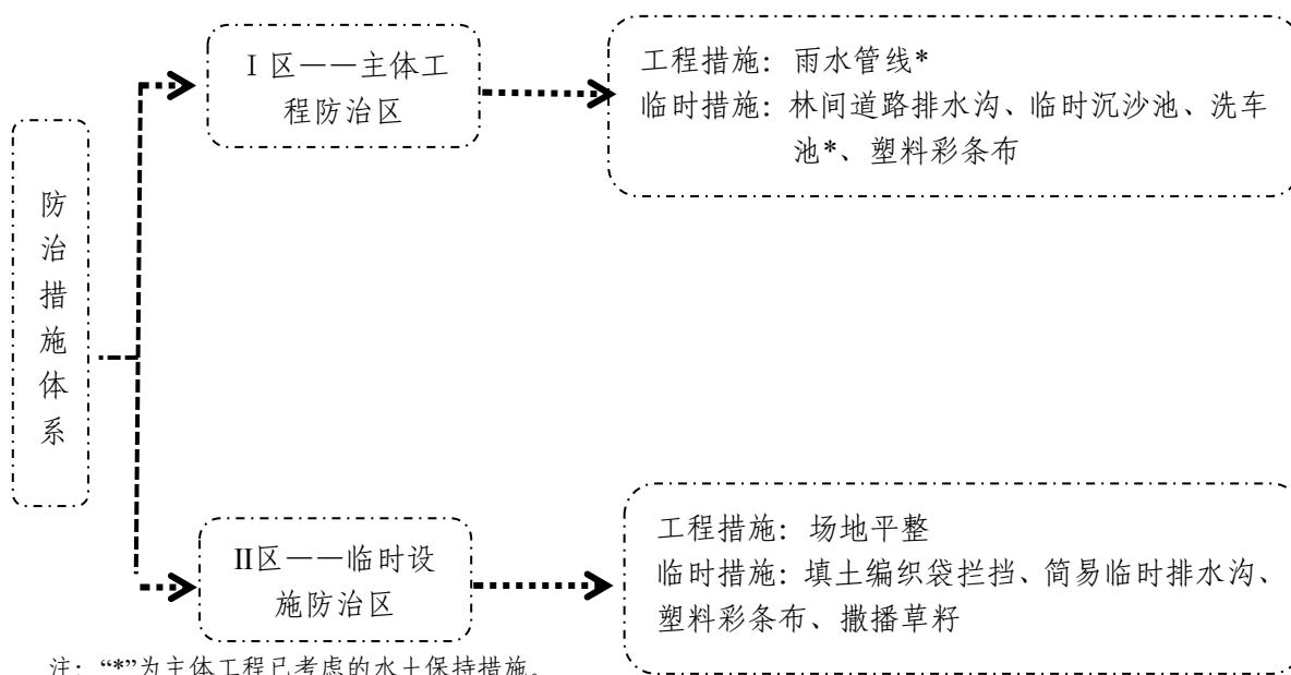
图 5-4 防治措施体系框图
