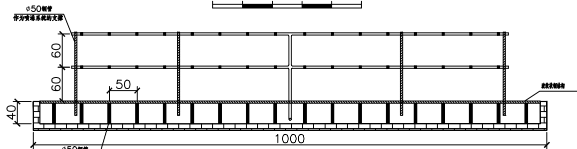
A-A'剖面图
