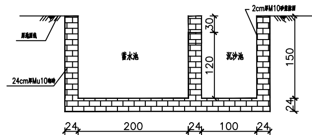
配套池体C-C'剖面图
