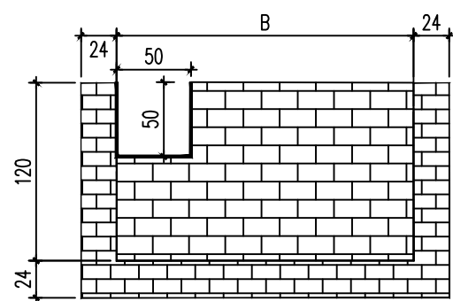
砖砌沉沙池B-B断面图 1:40
