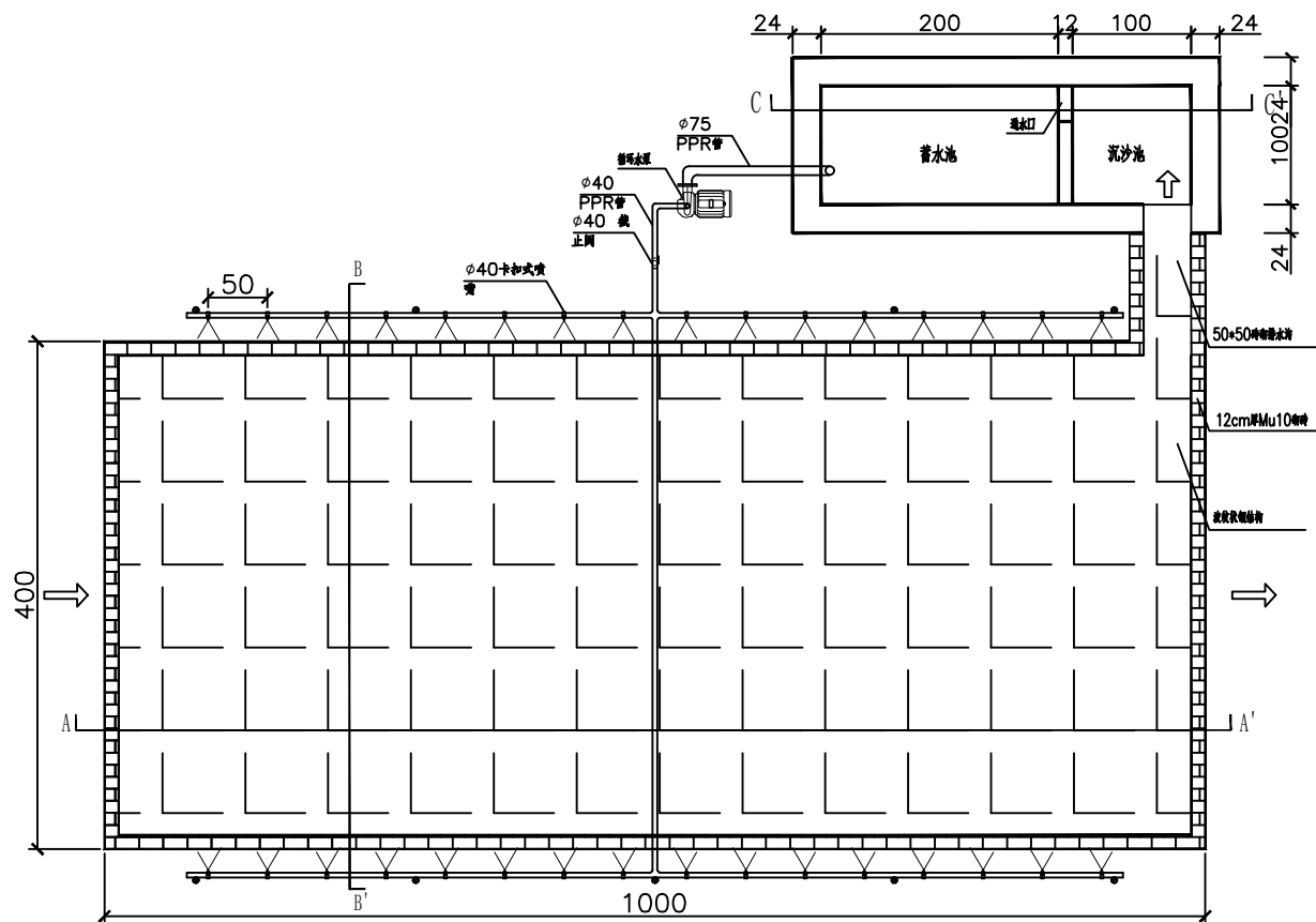
洗车池平面图
