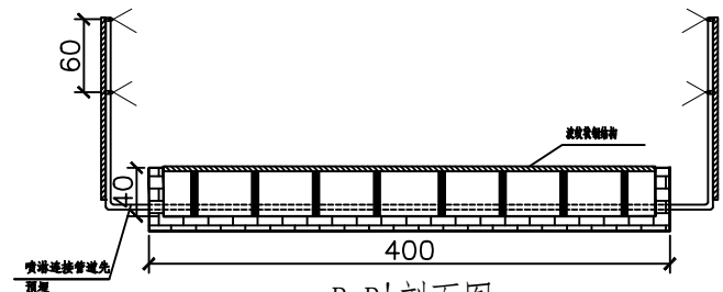
B-B'剖面图
