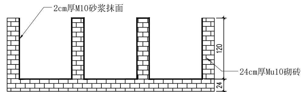
砖砌沉沙池A-A断面图 1:40
