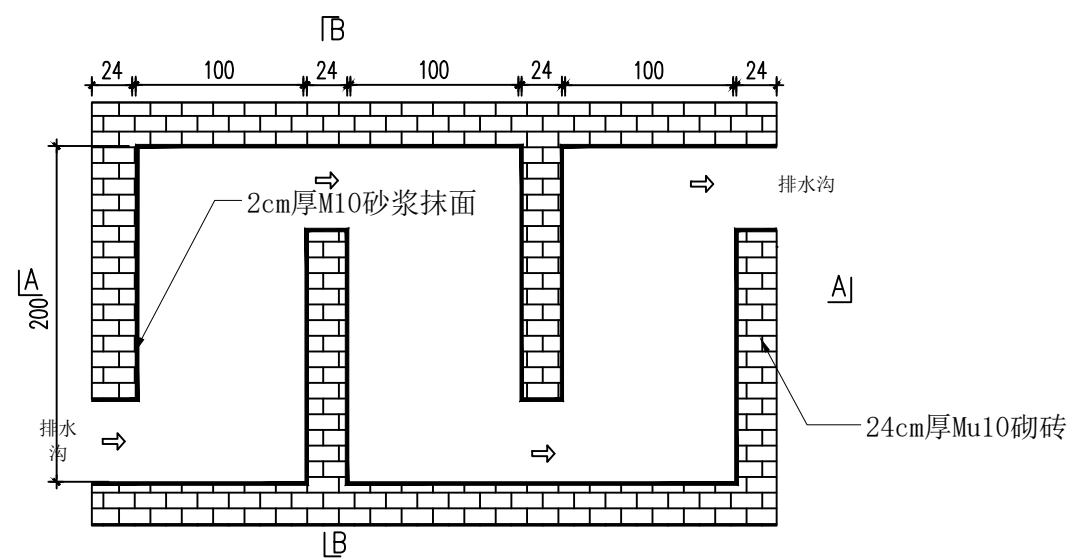
砖砌沉沙池平面布置图 1:40
