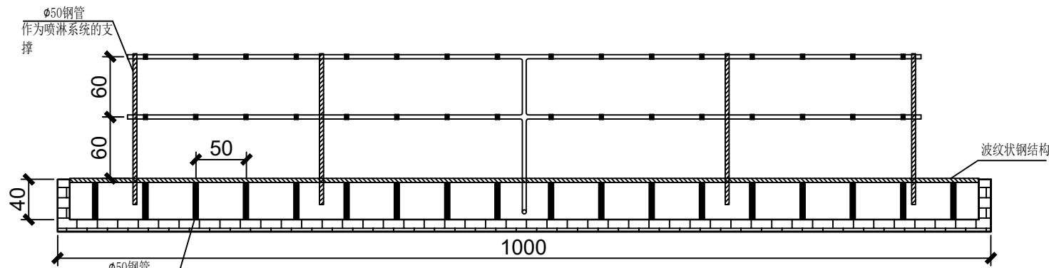
A-A'剖面图 1:50
