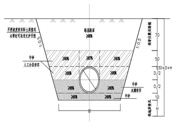
图 2-4 生产用水穿越青泰线典型开挖示意图
