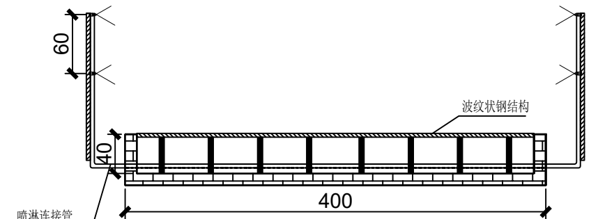
B-B'剖面图 1:50
