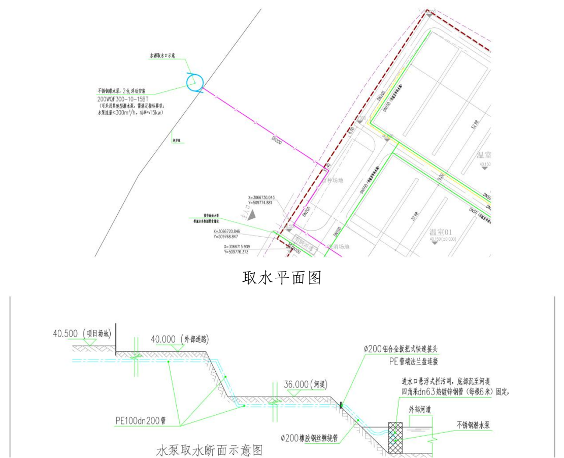
图 2-3 生产用水取水平面及断面示意图
