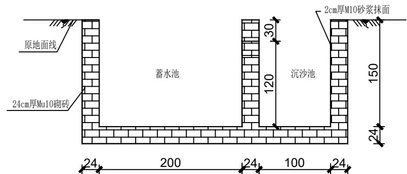
配套池体C-C'剖面图 1:50
